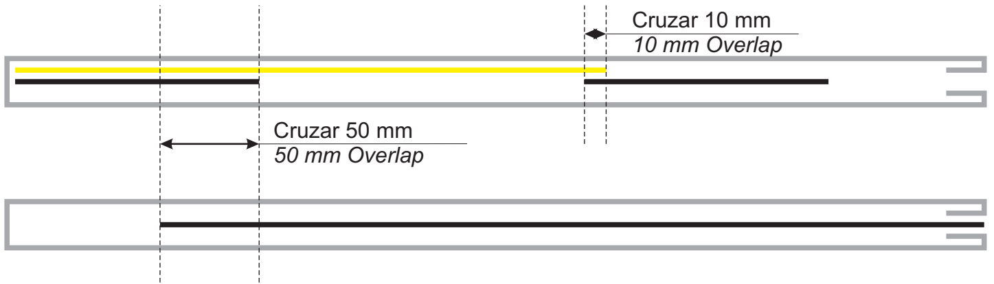
Colocación de la primera ala First wing attachment
