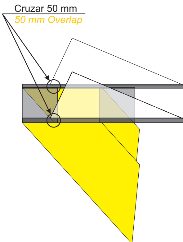
Colocación de las quillas Keels attachment
