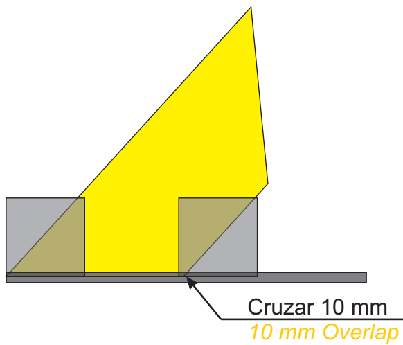
Colocación de la primera ala First wing attachment
